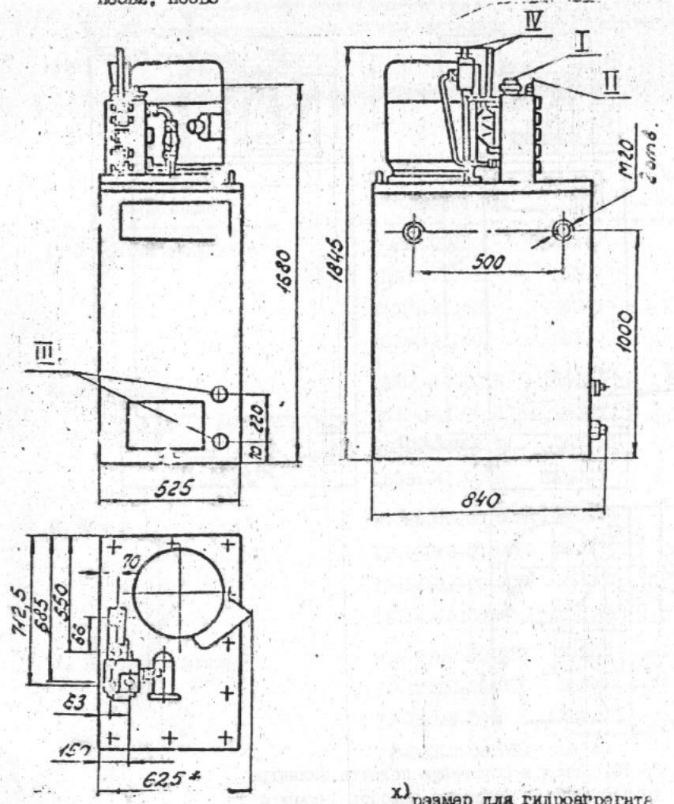
Рис. 2. Габаритные и присоединительные размеры гидроагрегатов П63В2, П63В3
