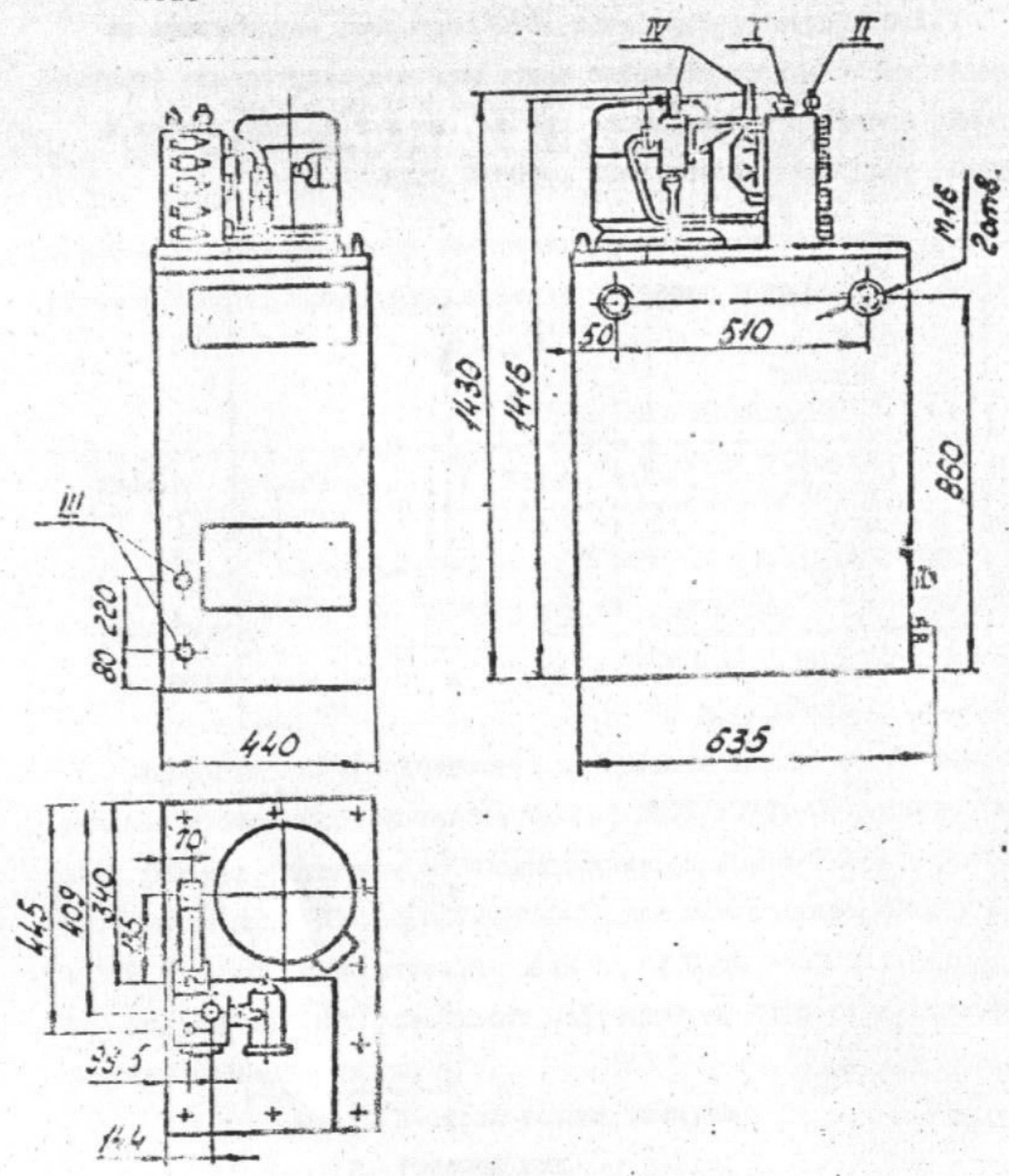
Рис. 1. Габаритные и присоединительные размеры гидроагрегата П63В1
