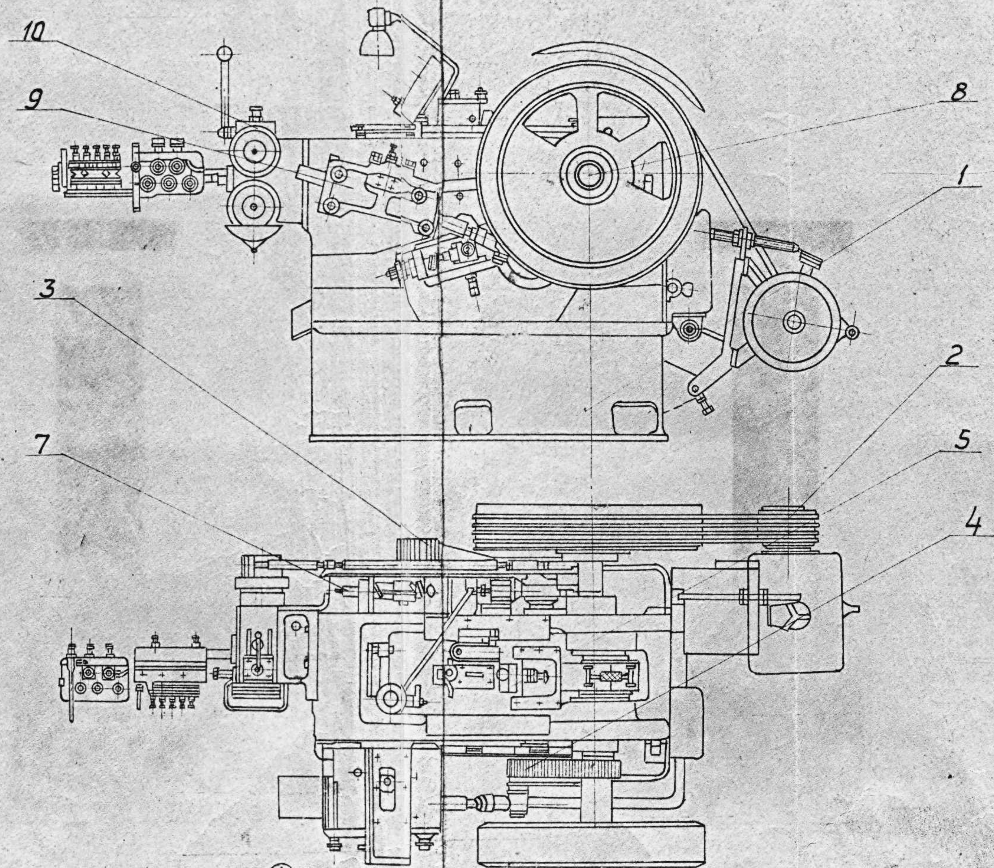
Рис. 2 ① Расположение основных частей автомата
