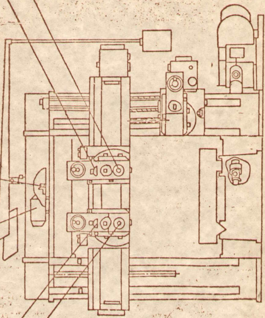
Рис. 11. Расположение электрооборудования на станке (Вид спереди)
