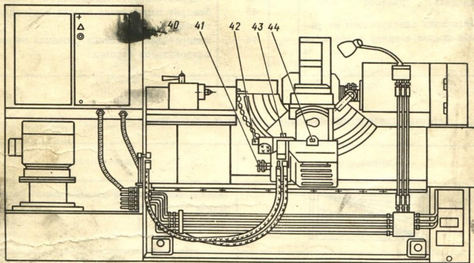
Рис. 2. Расположение органов управления на станке
