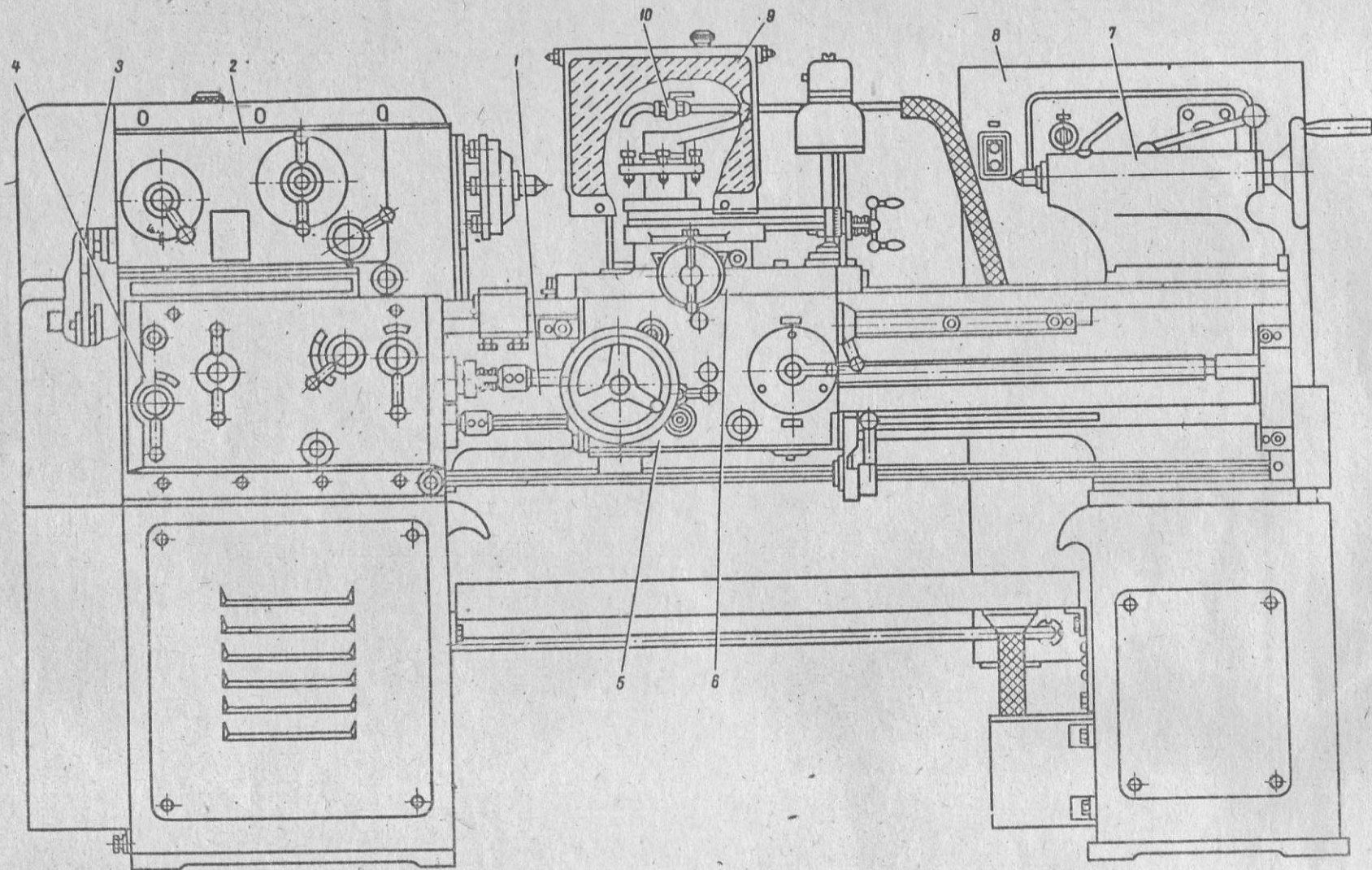
Рис. 2. Составные части станка
