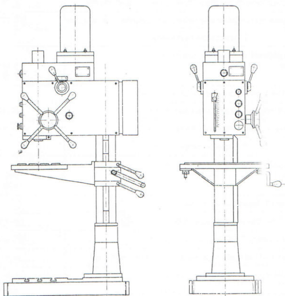
Рис.1. Общий вид станка
