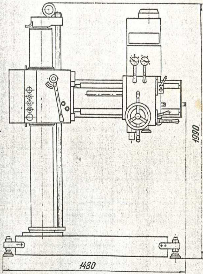
Рис. 1. Станок радиально-сверлильный
