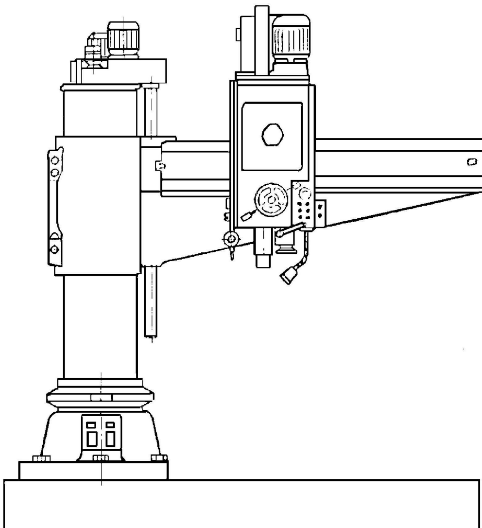
Рис. 1. Станок радиально-сверлильный модели 2М58-1
