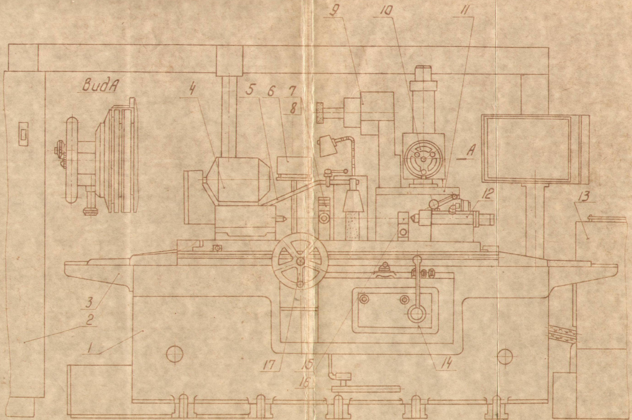
Рис. 2 Расположение составных частей станка.
