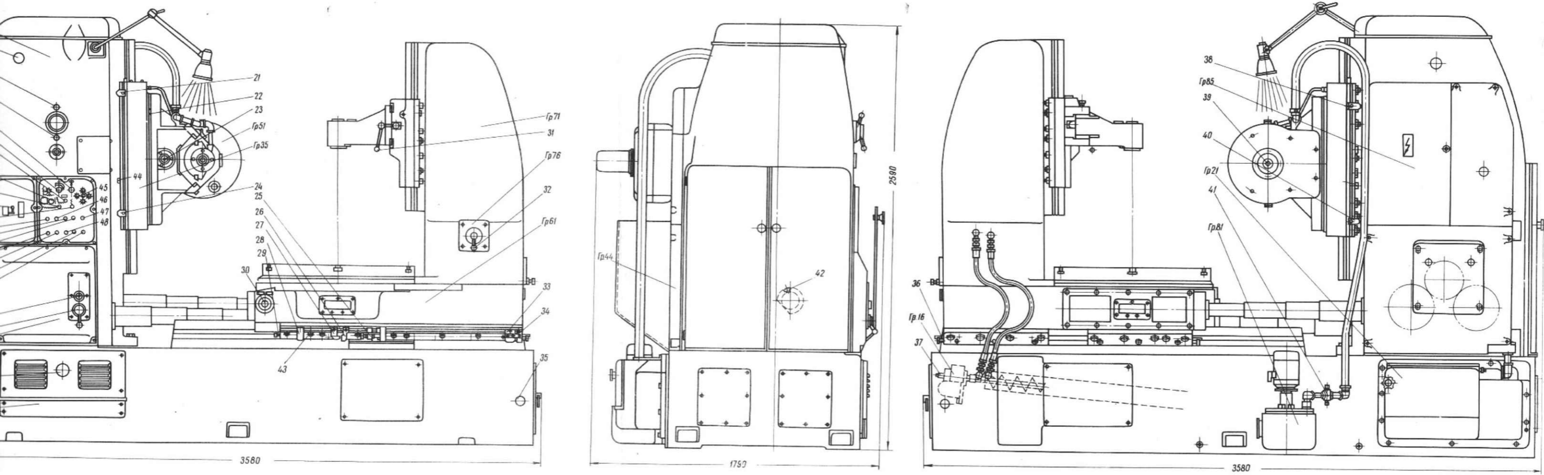
Рис. 4. Схема основных групп и органов управления станка
