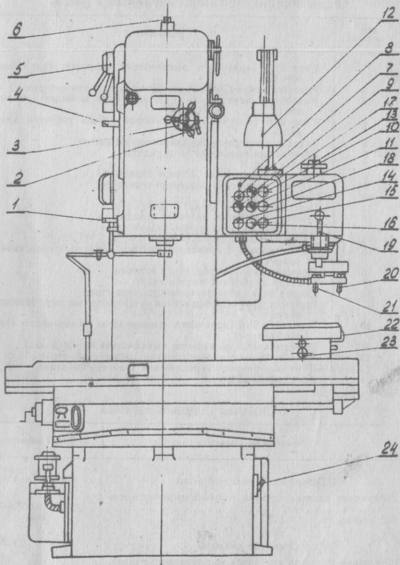
Рис. 3. Общий вид станка с обозначением органов управления.
