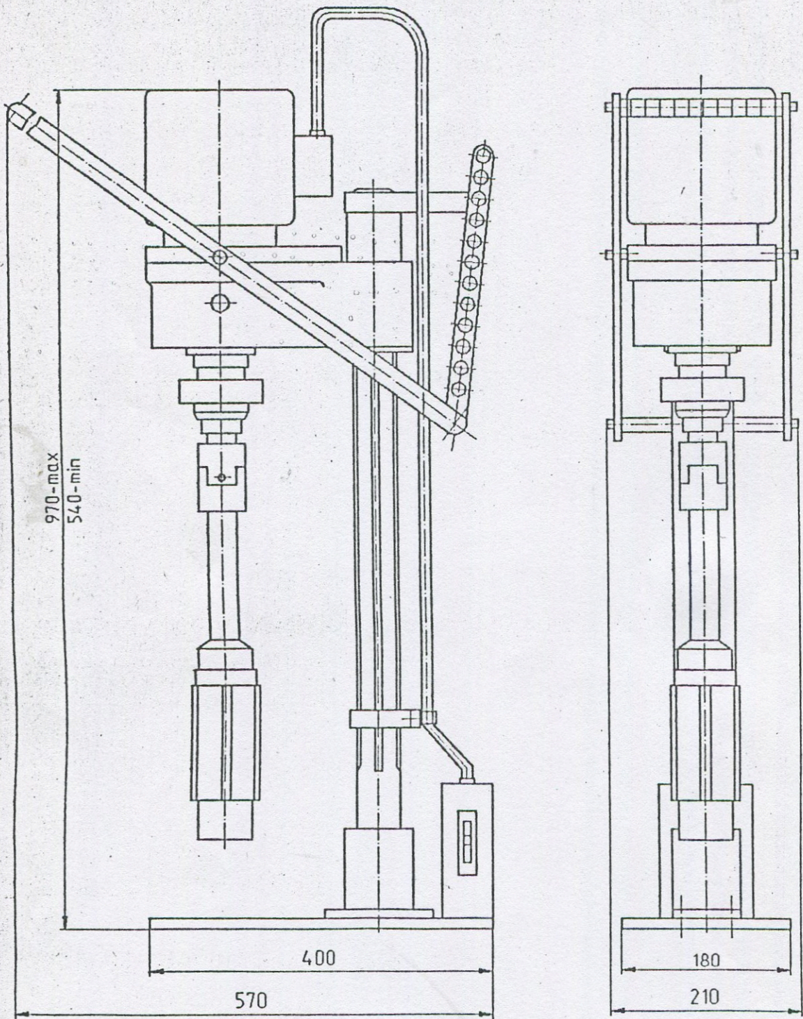
Рис.1. Общій вид станка
