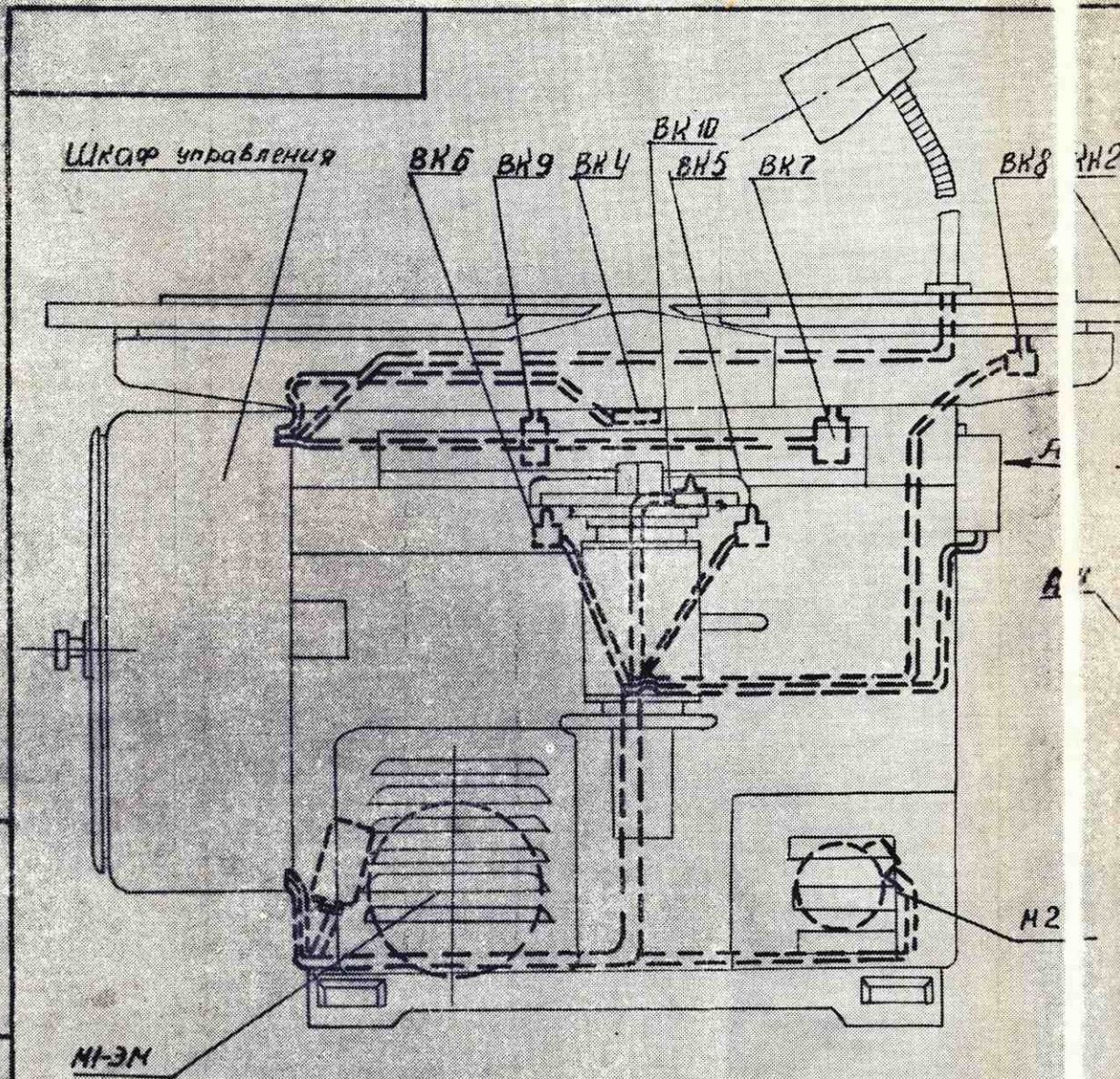
Вид А
