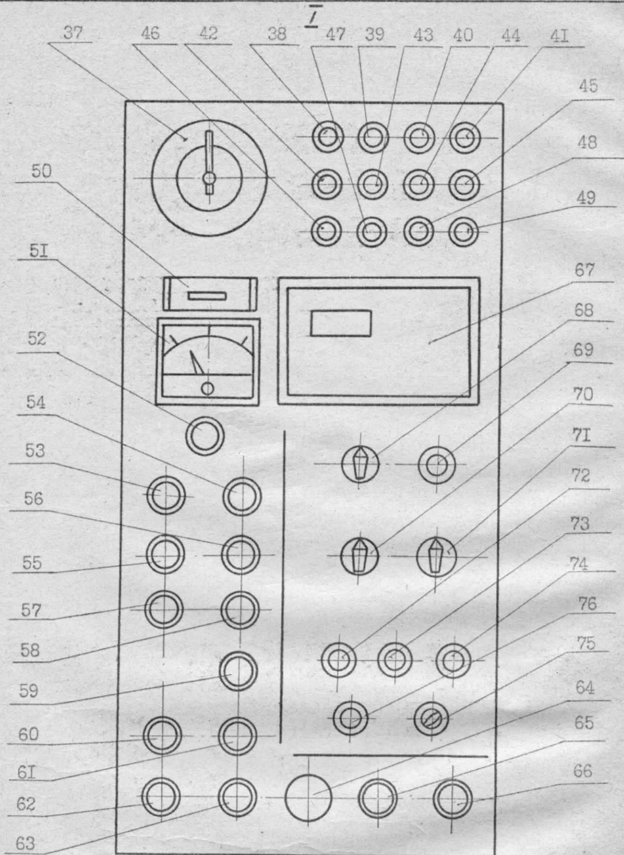
Рис. 6. Расположение органов управления, контролирующей и сигнализирующей аппаратуры на прессе (главный пульт)
