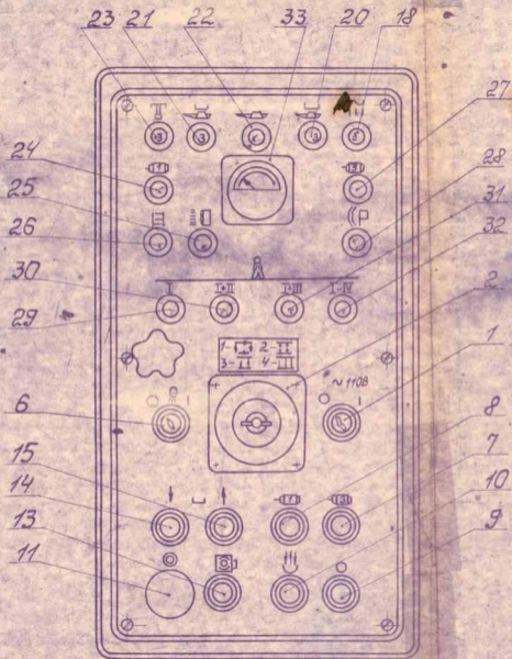
Рис. 1. ПАНЕЛЬ ПИТАНИЯ
