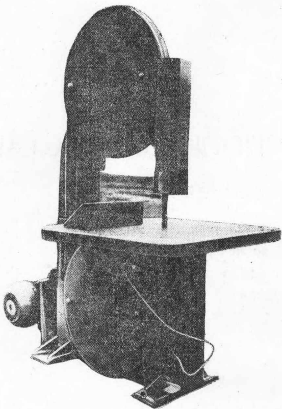
Рис. 1. Ленточнопильный станок, модель ЛС80-4.
