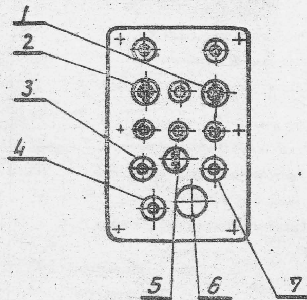
Рис. 2. Общий вид пульта управления с обозначением органов управления. 1 — переключатель «одиночный ход — автоматический ход», 2 — переключатель органов управления, 3 — кнопка «одиночный ход», 4 — кнопка «пуск» двигателя, 5 — выключатель цепи управления, 6 — кнопка «общий стоп», 7 — кнопка «стоп» автоматический ход.
