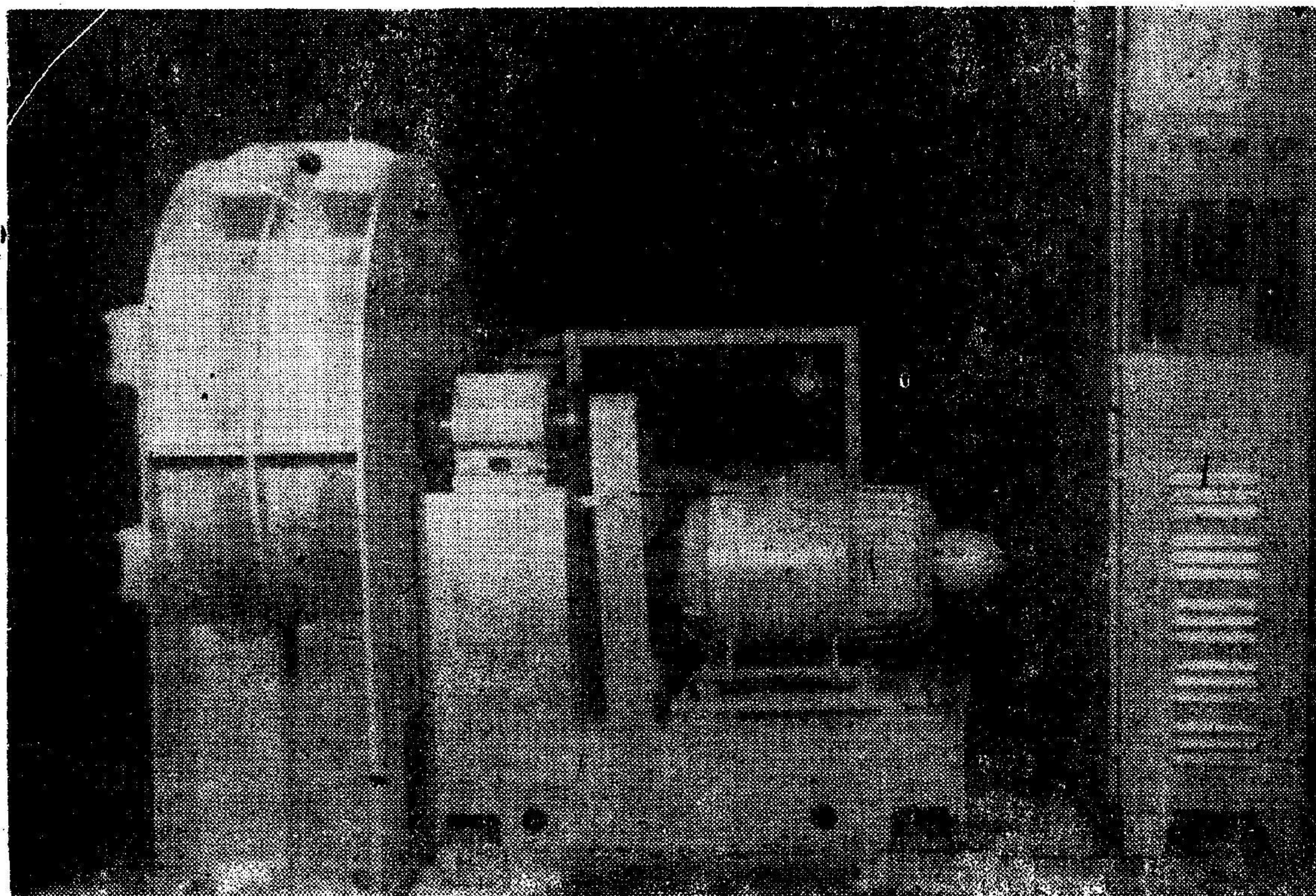
Станок однокамерный для испытания на прочность абразивных кругов.
