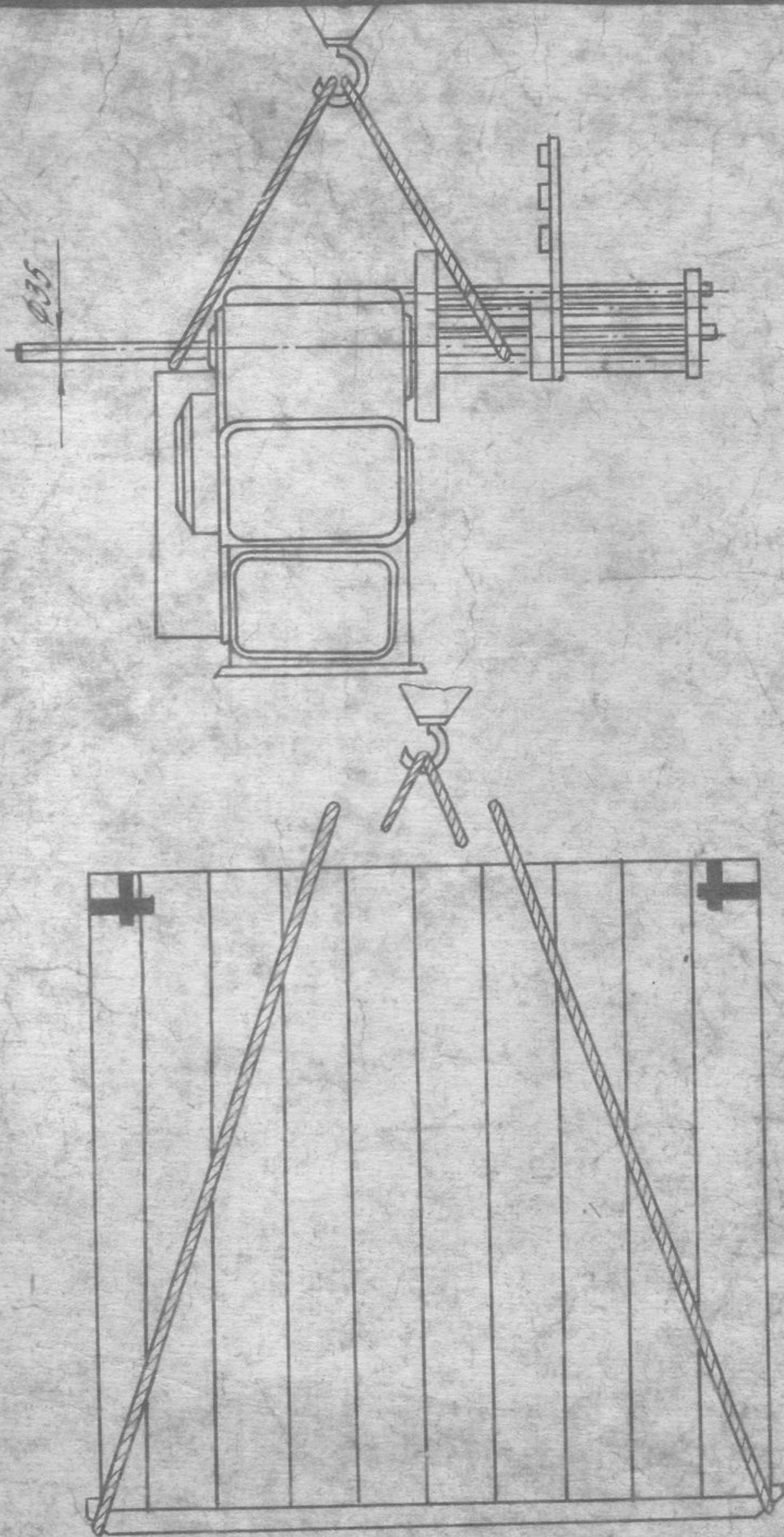
Схема транспортировки станка
